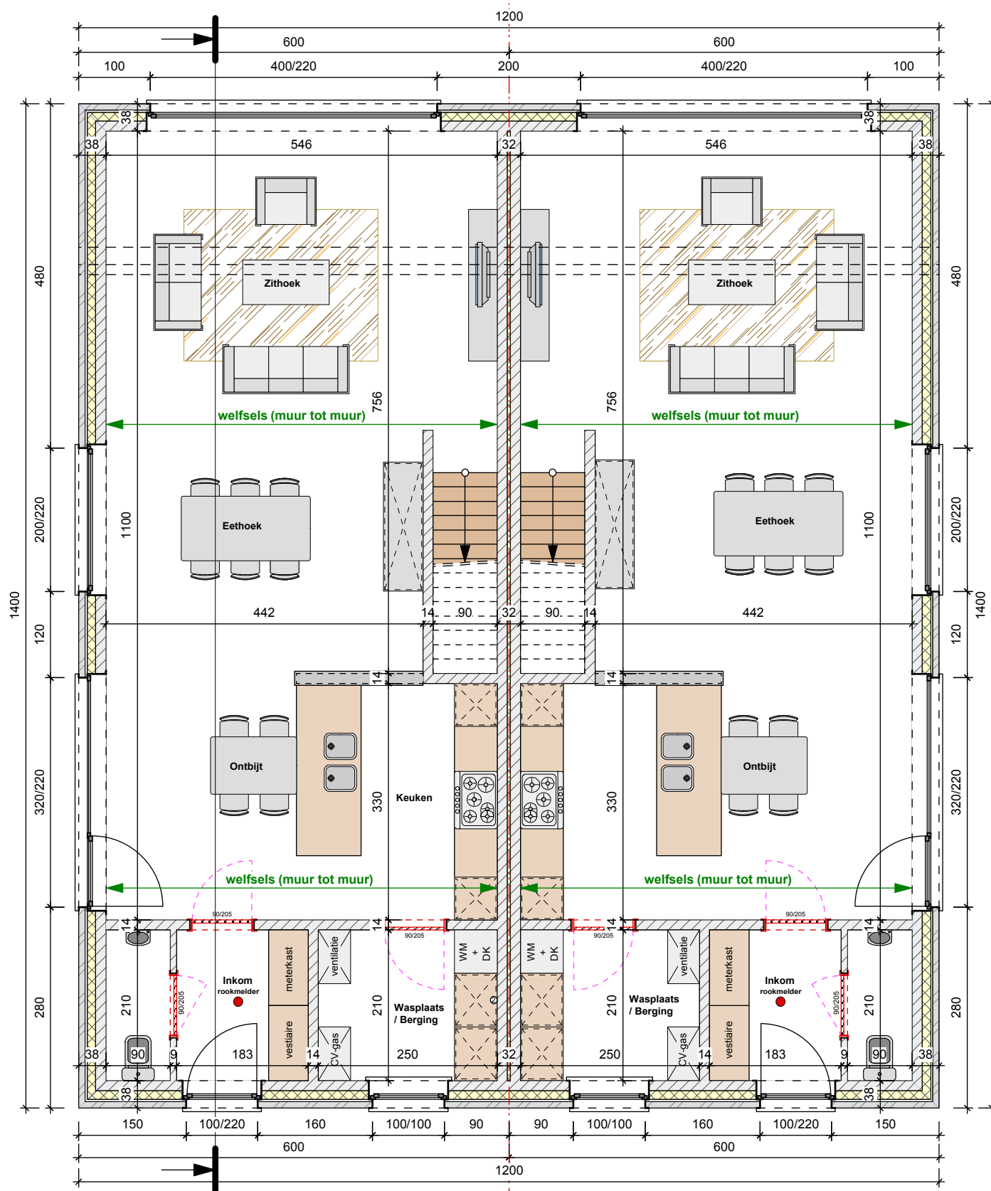
N Grondplan gelijkvloers schaal 1/75
