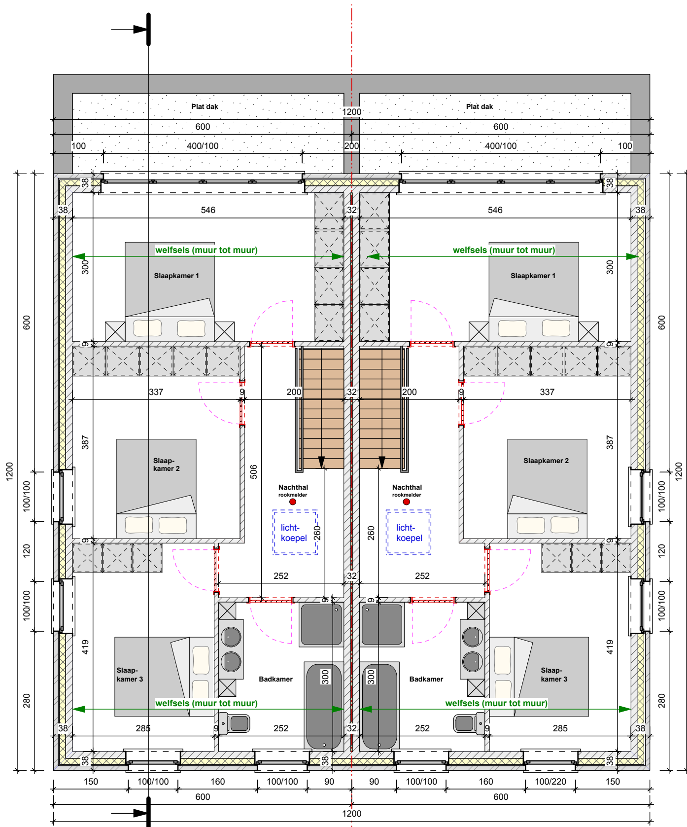
N Grondplan verdieping schaal 1/75
