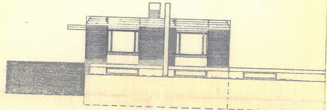
ZIJGEVEL RECHTS
