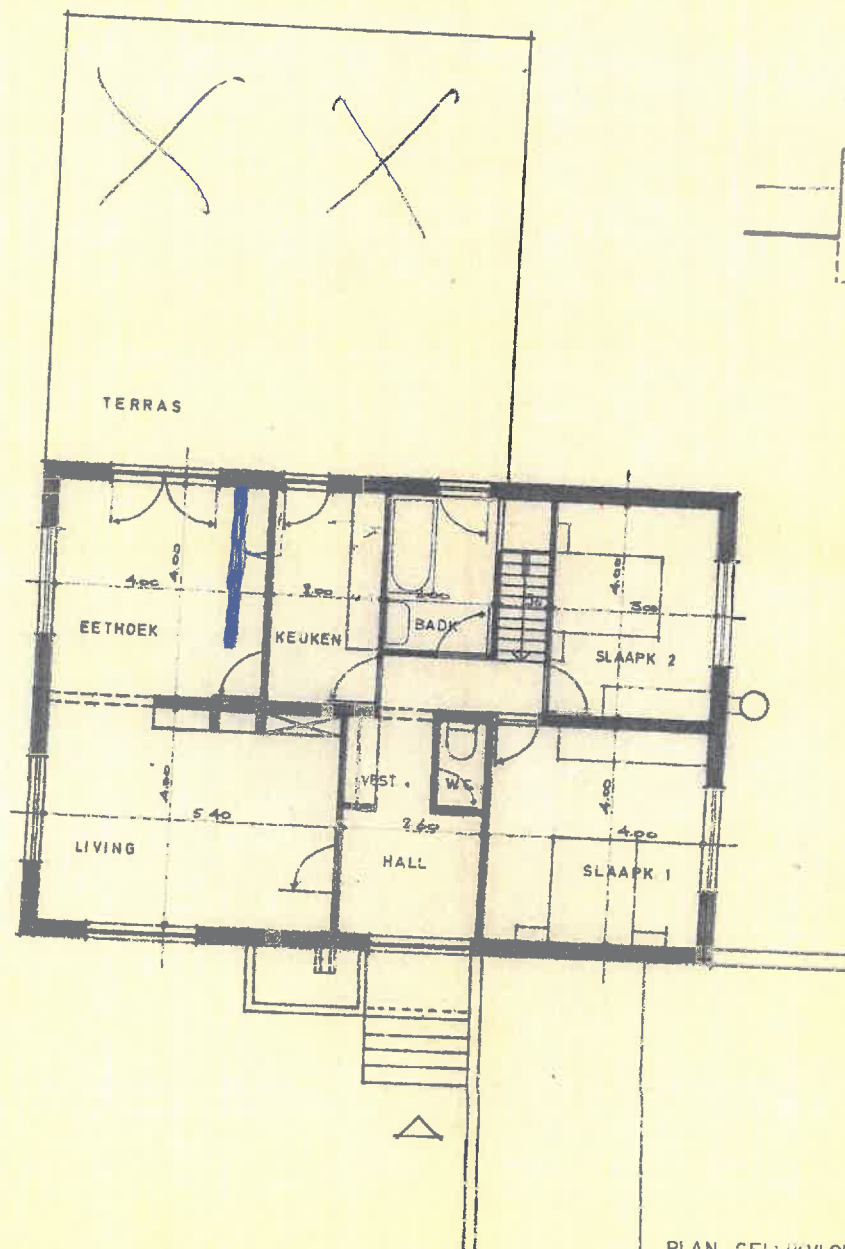
PLAN GELIJKVLOERS
